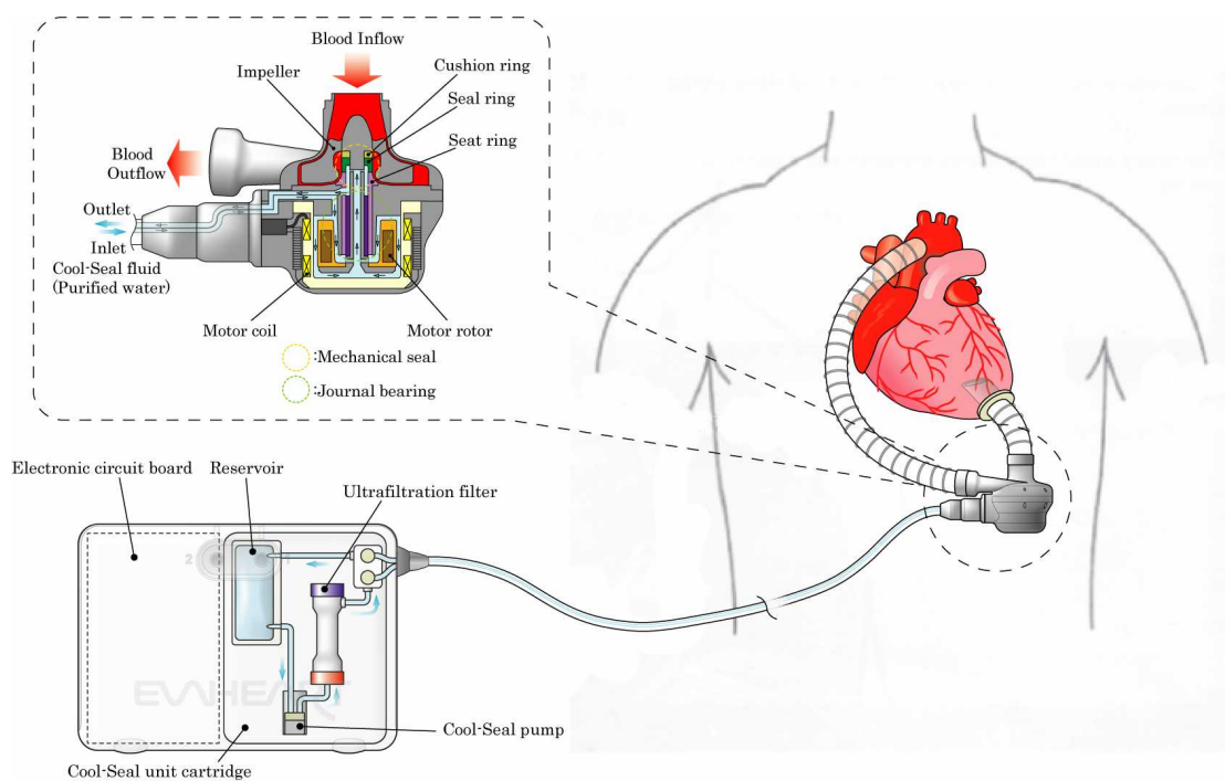
図 2 . EVAHEART のシェーマ。遠心ポンプは駆動ケーブルで体外携帯コントローラと接続されます。ポンプとコントローラ間で滅菌水が循環し、ポンプのジャーナルベアリングの潤滑モータコイル・メカニカルシールの冷却を行います。
